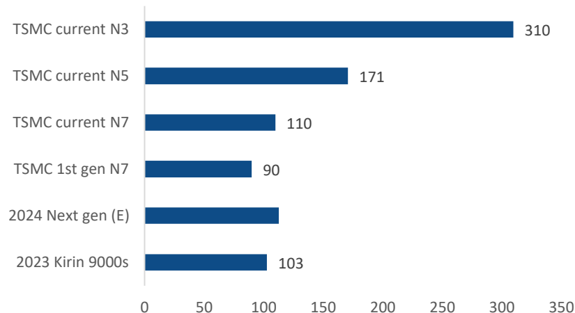
晶体管密度路标图 (mtr/mm 2 )
